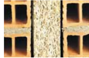
La separación entre paredes debe ser ligeramente superior al espesor del panel, para que éste pueda vibrar.
